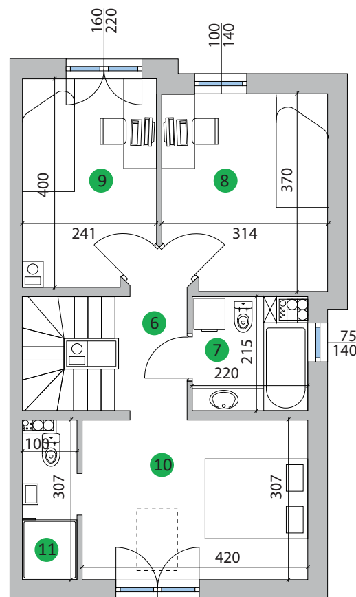
PIĘTRO 1
